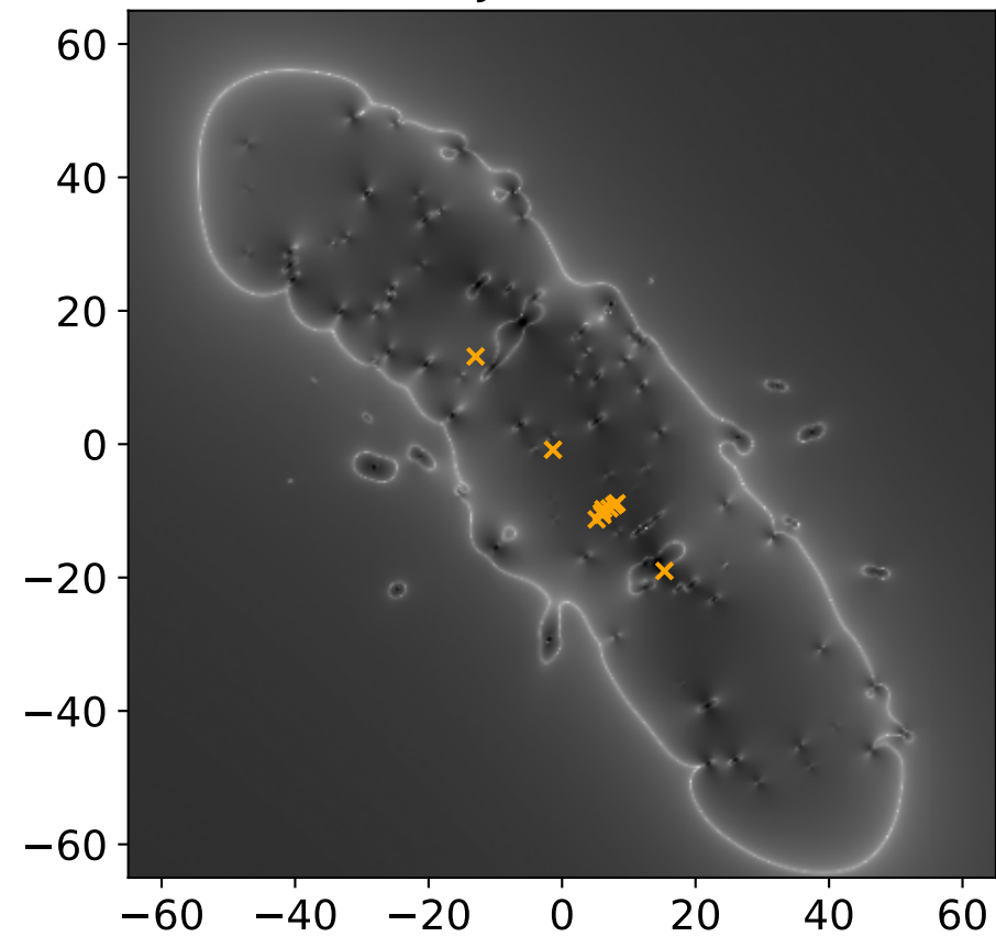
MACS J0416.1-2403
