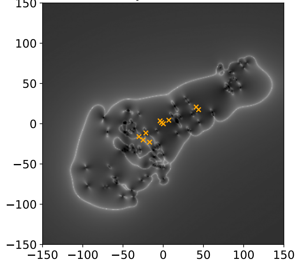
MACS J0717.5+3745
